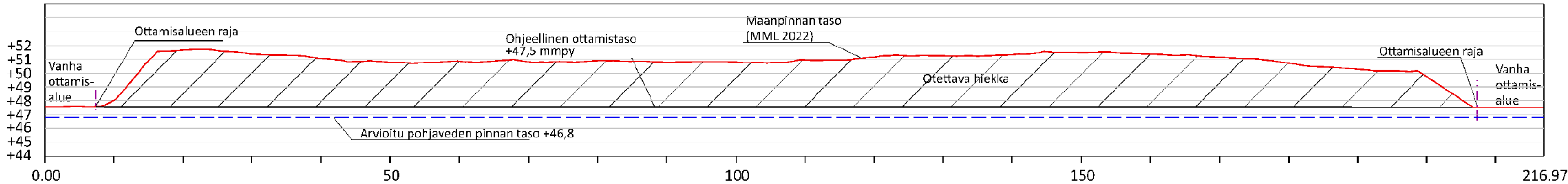
LEIKKAUS B - B mk 1:1000 / 1:500
