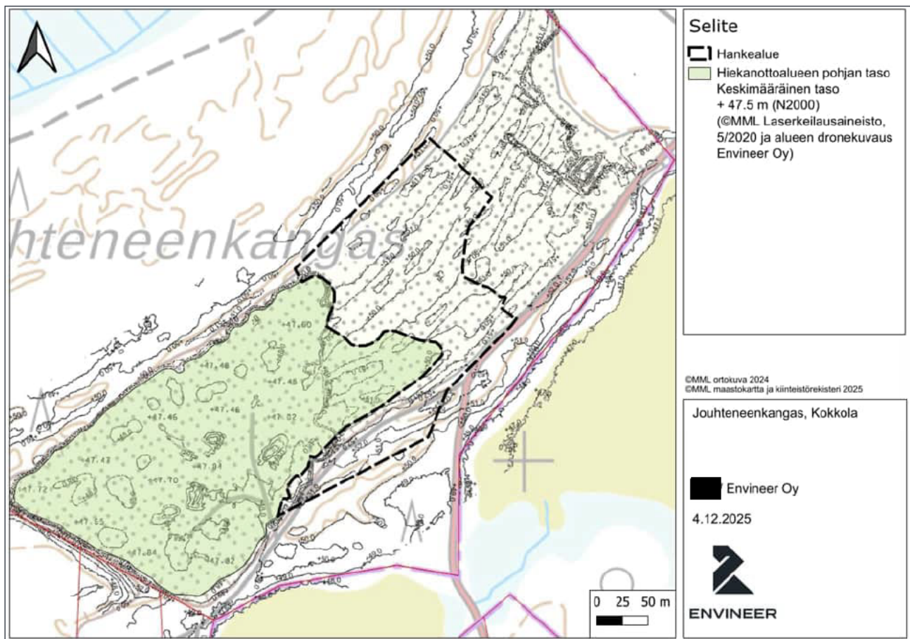
Kuva 4. Ottoalueen korot (MML Laserkeilausaineisto 5/2020).
