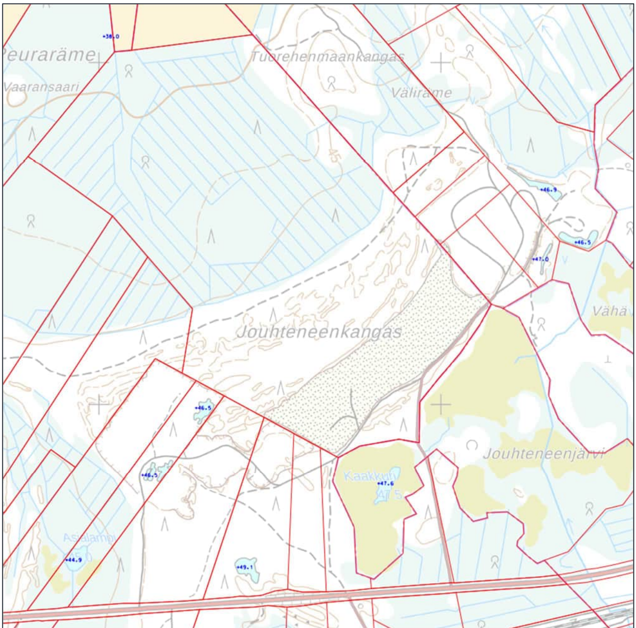
Kuva 7. Ottoalueen lähiympäristön pintavesien korot (MML Laserkeilausaineisto 5/2020).
