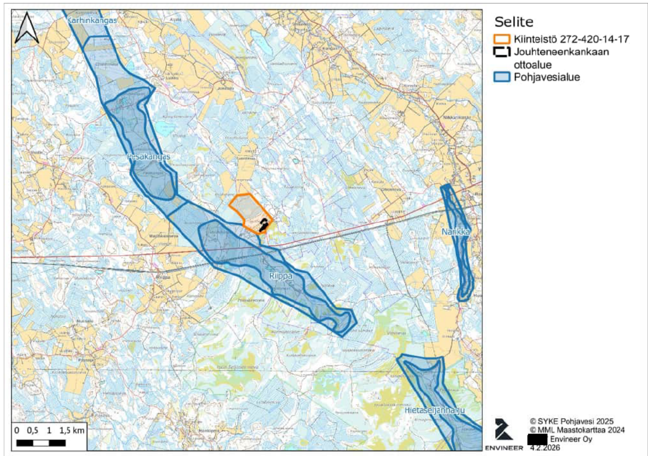
Kuva 8. Kiinteistö 272-420-14-17, Jouhteneenkankaan ottoalue ja lähimmät pohjavesialueet.
