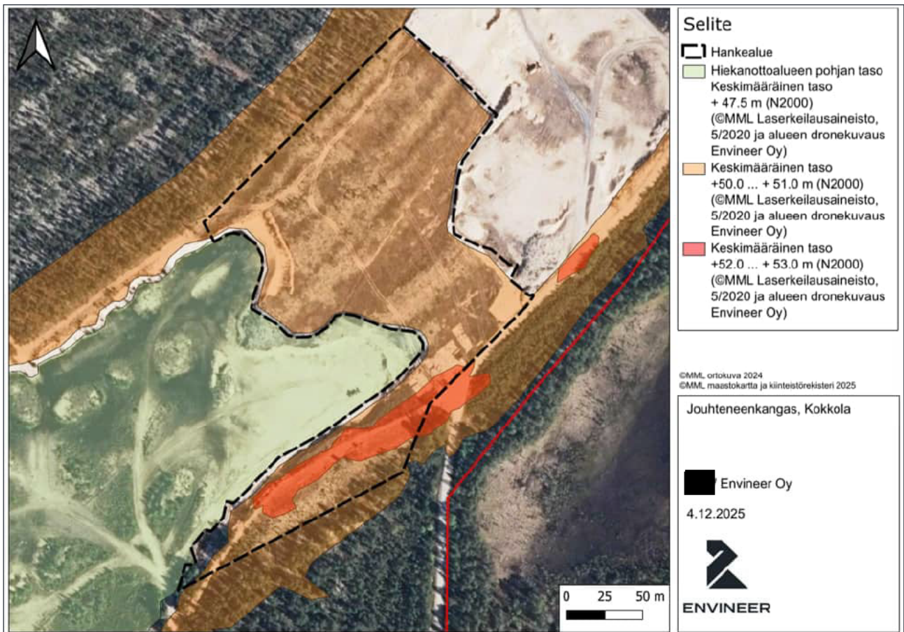
Kuva 6. Nykytilanne ja suunniteltu otto (MML Laserkeilausaineisto).
