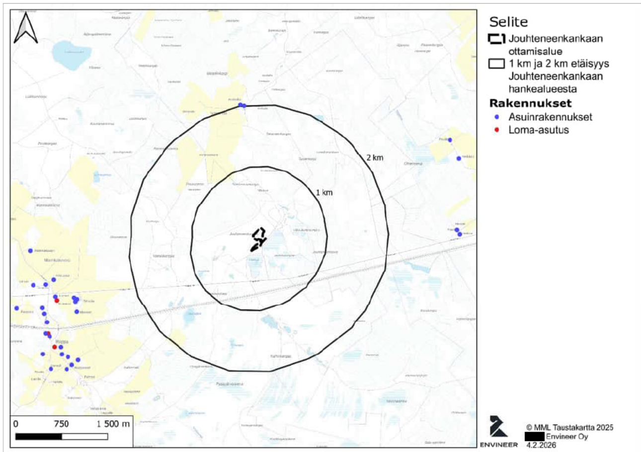
Kuva 3. Asuinrakennukset ja loma-asutus.
