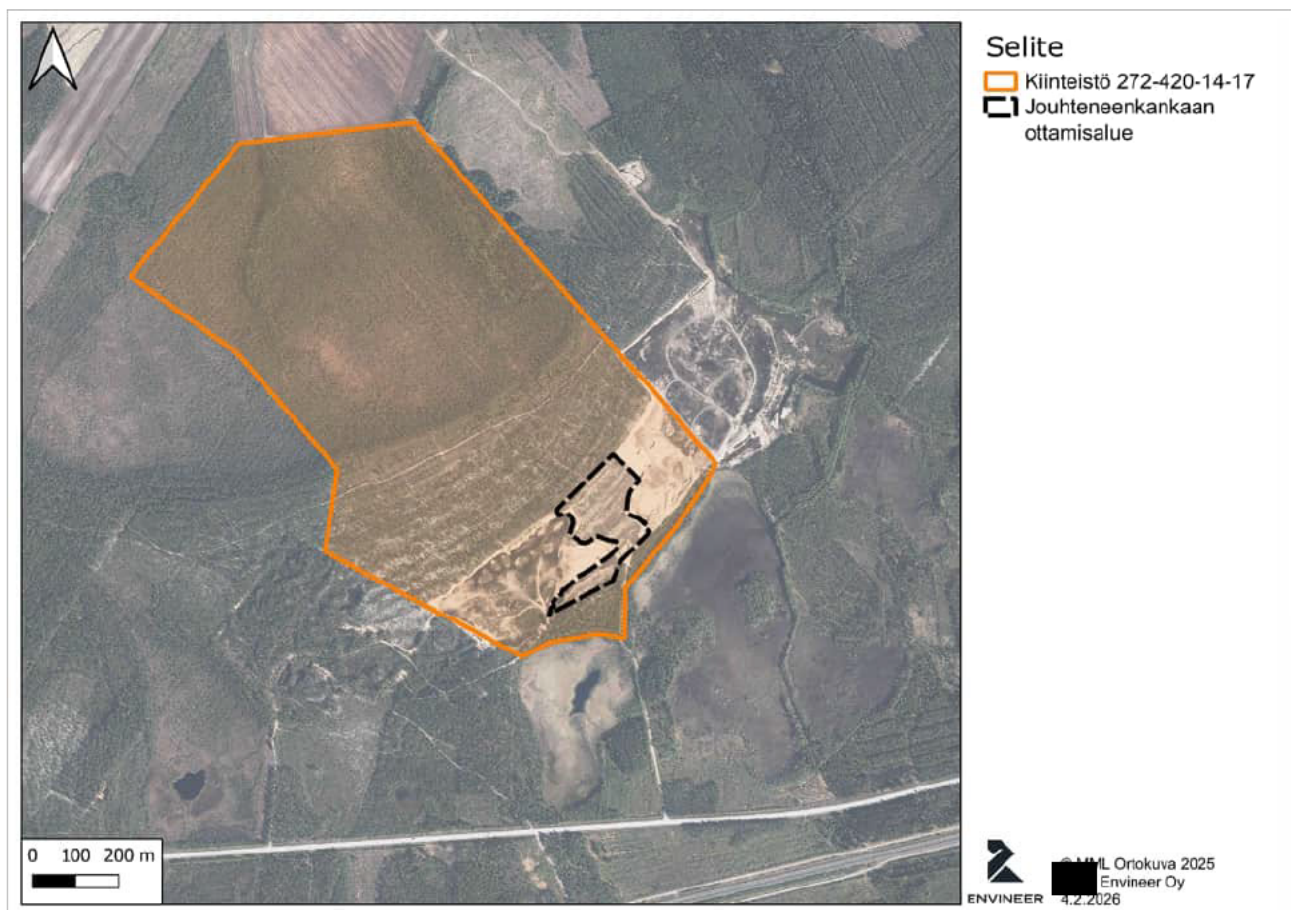
Kuva 2. Kiinteistö 272-420-14-17 ja ottoalue.
