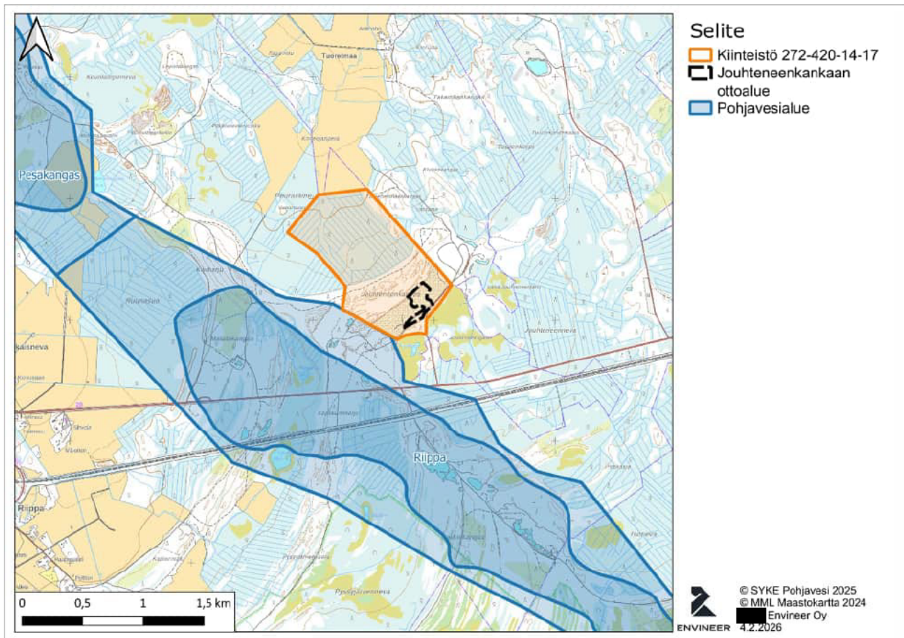
Kuva 9. Kiinteistö 272-420-14-17, Jouhteneenkankaan ottoalue ja lähimmät pohjavesialueet.
