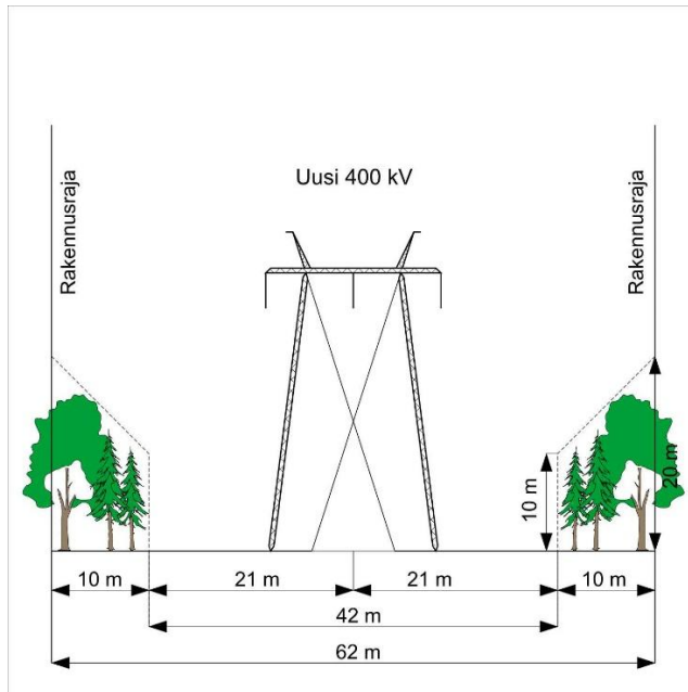
Kuva 7. Hankkeessa arvioitava 400 kV johdon pylvästyyppi ja johtoalueen leveys.
