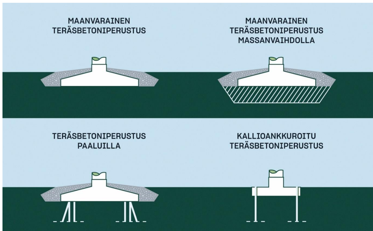
Kuva 4. Tuulivoimaloiden perustamistekniikoita (OX2 2022).
