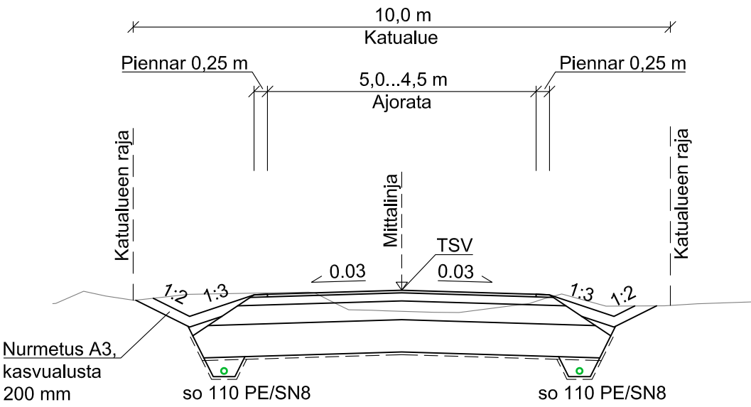
POIKKILEIKKAUS A - A 1:100
